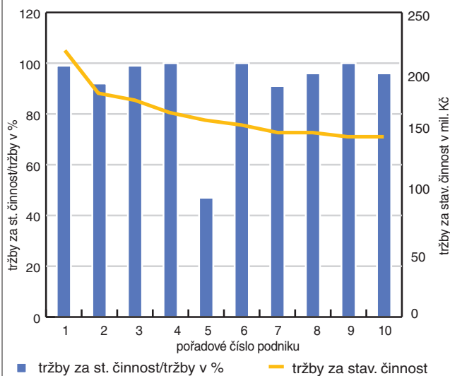
TOP 10 podniků podle velikosti tržeb za stavební činnost
